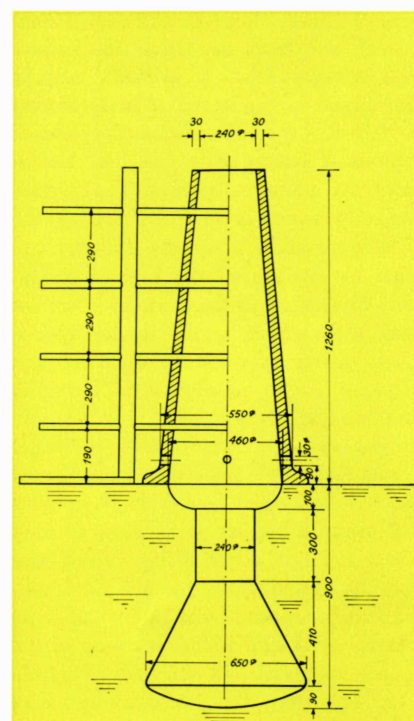
Fig. 1 Snit gennem Drenghsted-ovnen efter magister Olfert Voss' rekonstruktionsforslag. Stativet til venstre i billedet bærer temperaturmåleinstrumenterne.
