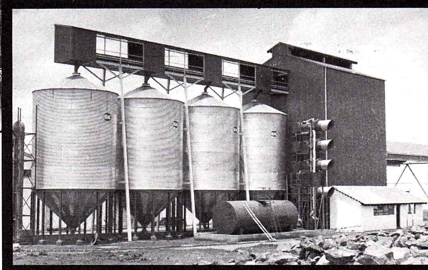
Majsanlæg til Kenya. Maize plants for Kenya.
