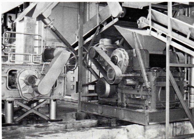
Hammermølle (til højre) og valse Hammermill (right) and creper ▼
