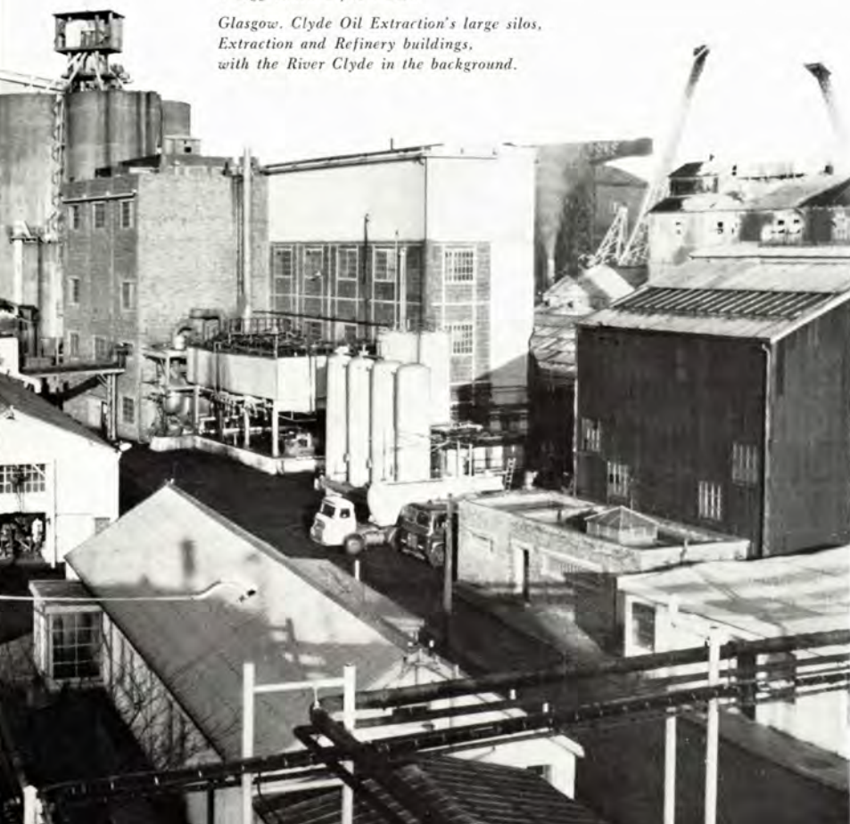
Glasgow. Clyde Oil Extractions store siloer, Ekstraktionsbygning og Raffinaderi. I baggrunden Clyde-floden.
